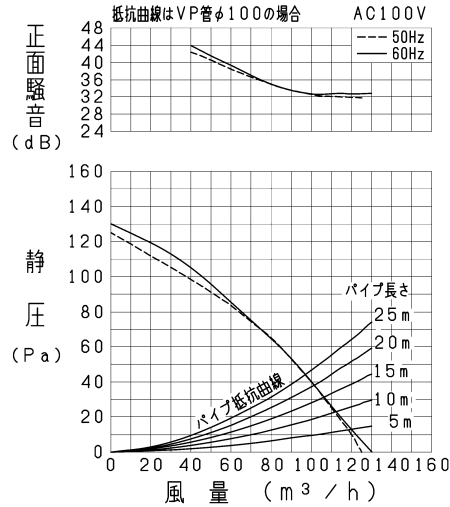
VD-13ZC 1.4 -IN/P-Q・騒音特性
