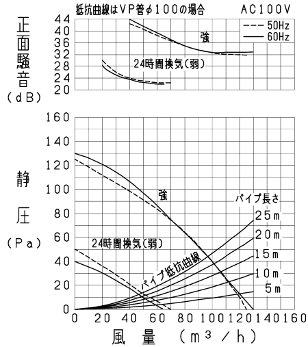
VD-13ZLC 1.4 -IN/P-Q・騒音特性
